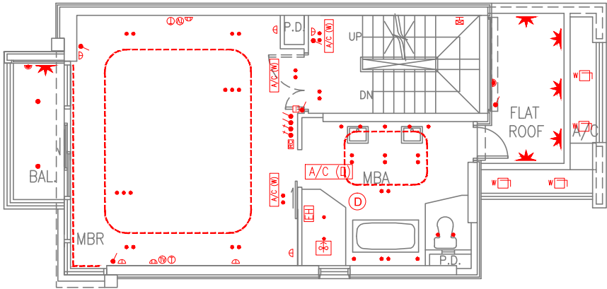
HOUSE LEVEL 3 PLAN 獨立屋第三層平面圖
