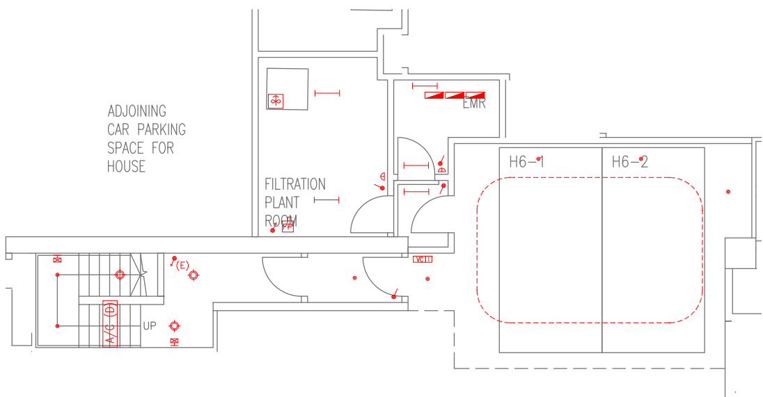
HOUSE CARPARK LEVEL PLAN 獨立屋停車層平面圖
