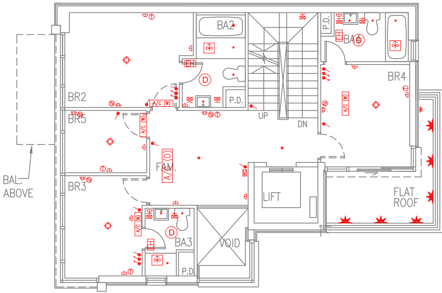
Mechanical & Electrical Provisions Plan 機電裝置平面圖
